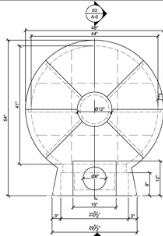
01 OVEN PLAN A-0 SCALE: 3/4"=1'-0"
