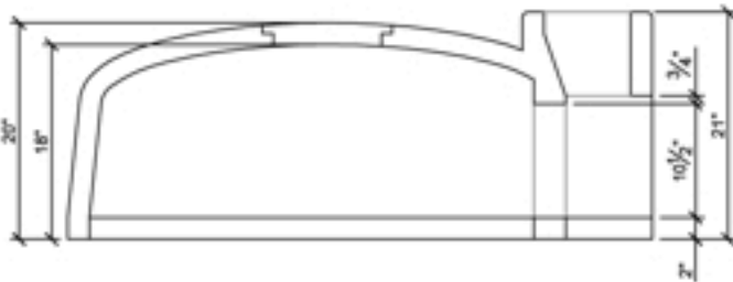
03 SIDE ELEVATION A-0 SCALE: 3/4"=1'-0"
