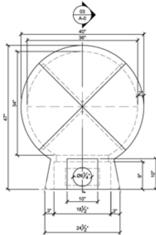
01 OVEN PLAN A-0 SCALE: 3/4"=1'-0"
