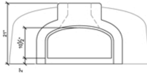
02 FRONT ELEVATION A-0 SCALE: 3/4"=1'-0"
