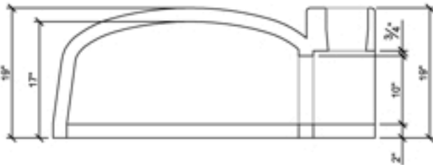
03 SIDE ELEVATION A-0 SCALE: 3/4"=1'-0"
